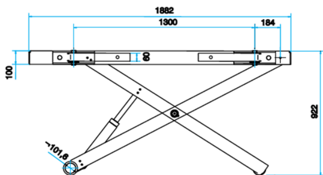
STL29 with set of wheels - avec kit de roues
