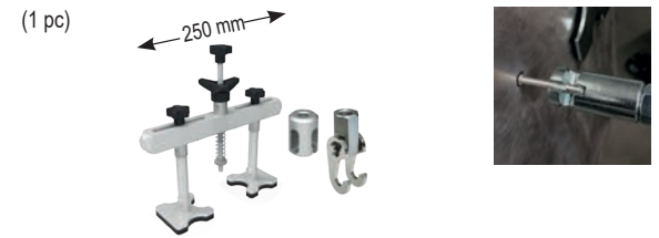
011044 250 mm Traversa Levelling bar
