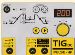
MASTROTIG 218 DC
