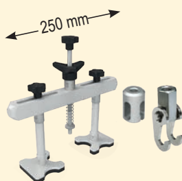
011044 250 mm (1 pc)
