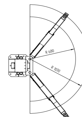
OPTIONAL VERSION - DOUBLE EXTENSION ARM OPTIONAL VERSION - BRACCI A DOPPIO SFILLO
